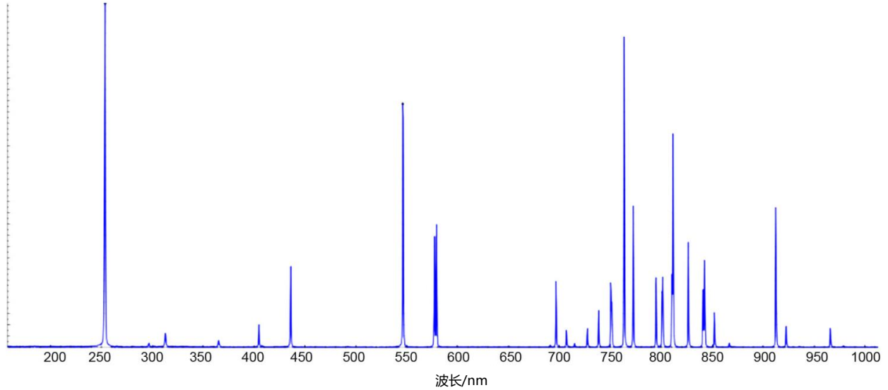
200~1000nm测试结果和应用——汞灯光谱
