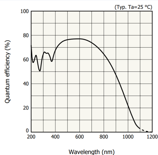
CCD量子效率曲线
